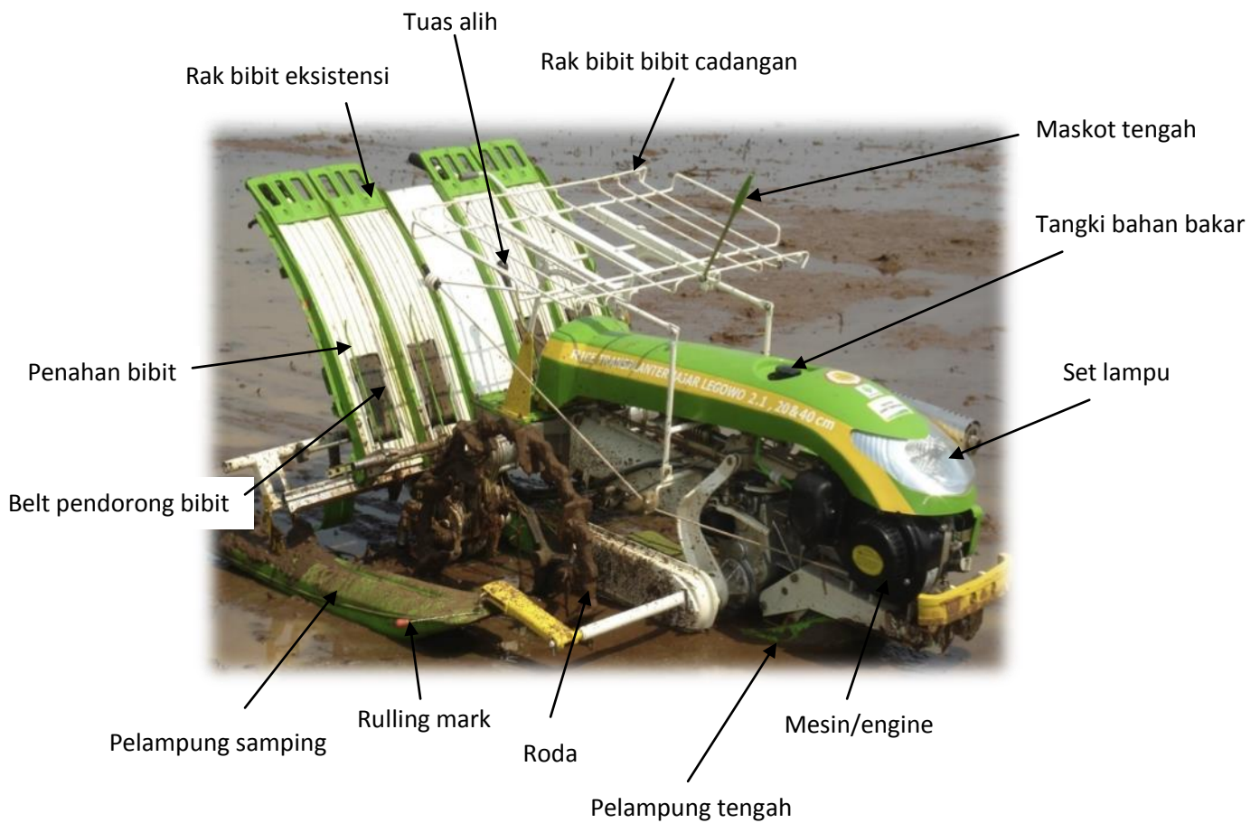
Gambar 1. Bagian-bagian Depan Mesin Transplanter
