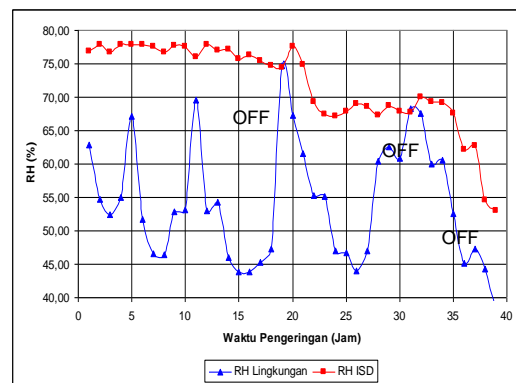
Gambar 11. Fluktuasi RH selama pengeringan pada pengujian 2
