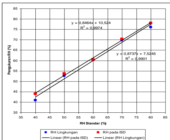
Gambar 6. Nilai hasil kalibrasi RH sensor SHT75 dengan alat pengeringan
