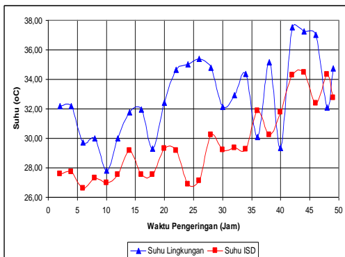
Gambar 8. Fluktuasi suhu selama pengeringan pada pengujian 1
