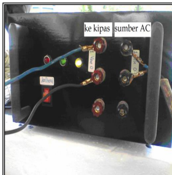
Gambar 3 Perangkat sistem kendali tampak luar
