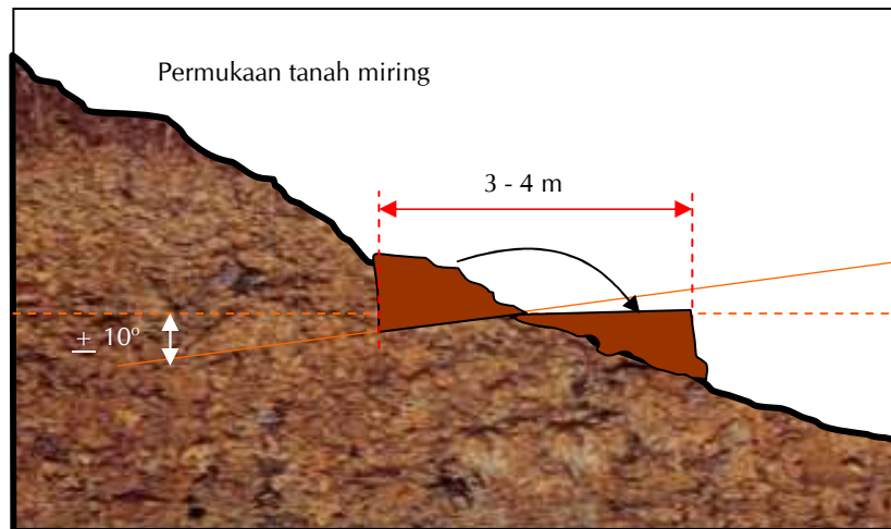
Gambar 9. Skema bentuk teras bangku
