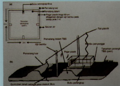
Gambar 3. Skema pemasangan TBS, Tampak atas (a), letak pemasangan komponen TBS (b)
