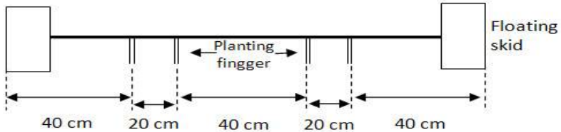
Gambar 3. Ukuran dan posisi jarak jarwo pada Indojaro transplanter
