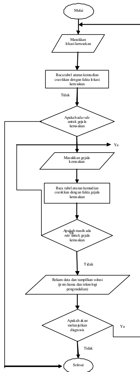
Gambar 6. Algoritma Mesin Inferensi.
