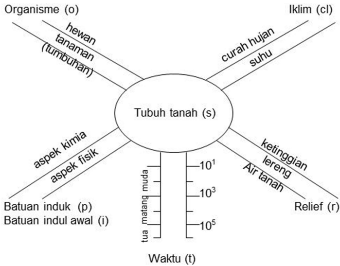
Gambar 6. Diagram faktor-faktor pembentuk tanah.
