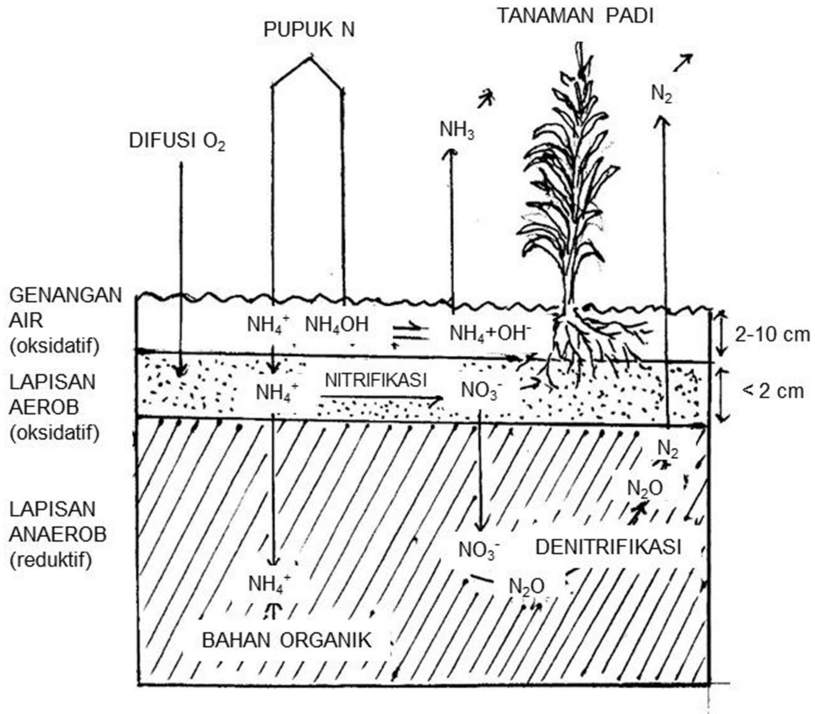
Gambar 13. Transformasi pupuk N menjadi gas \text{NH}_3 dan \text{NH}_4^+ menjadi \text{NO}_3^- di lapisan oksidasi (nitrifikasi) dan \text{NO}_3^- menjadi \text{N}_2\text{O} dan \text{N}_2 di lapisan reduksi (denitrifikasi).
