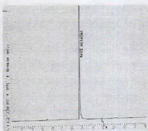
Gambar 1 Kromatogram minyak gandapura jenis daun lebar ( G. fragrantissima )
