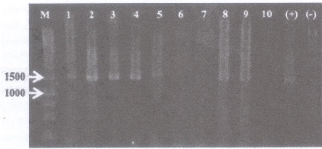
Gambar 1. Visualisasi amplifikasi sebagian gen selubung protein RTBV dengan PCR menggunakan primer RTBV-DA F dan RTBV DA R.
