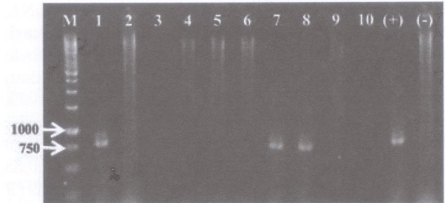
Gambar 2. Visualisasi amplifikasi sebagian gen selubung protein RTSV dengan RT-PCR menggunakan primer RTSV-F2 dan RTSV-R2.
