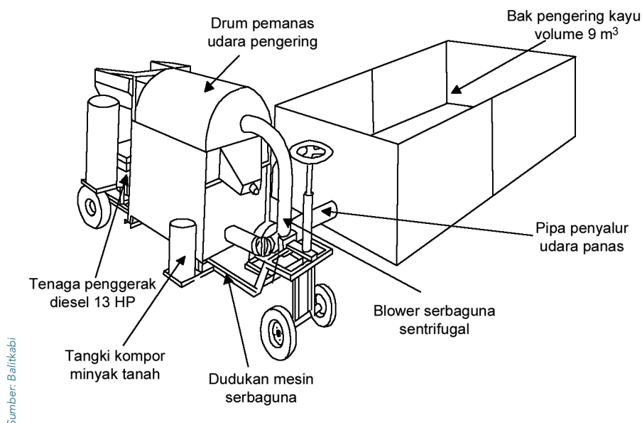
Prototipe alat pengering kedelai brangkasan tipe bak
