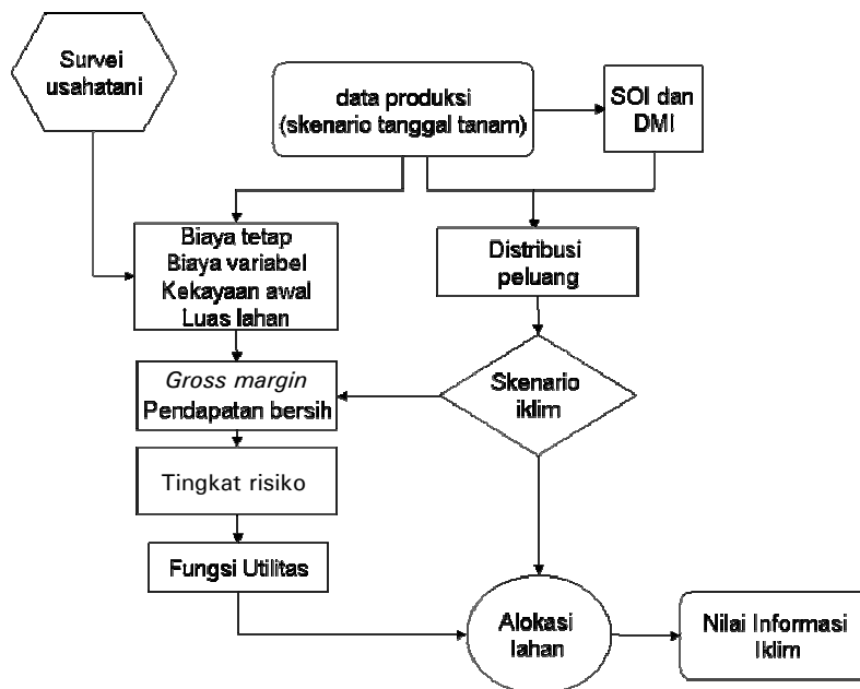
Gambar 1. Tahapan analisis pemanfaatan informasi iklim
