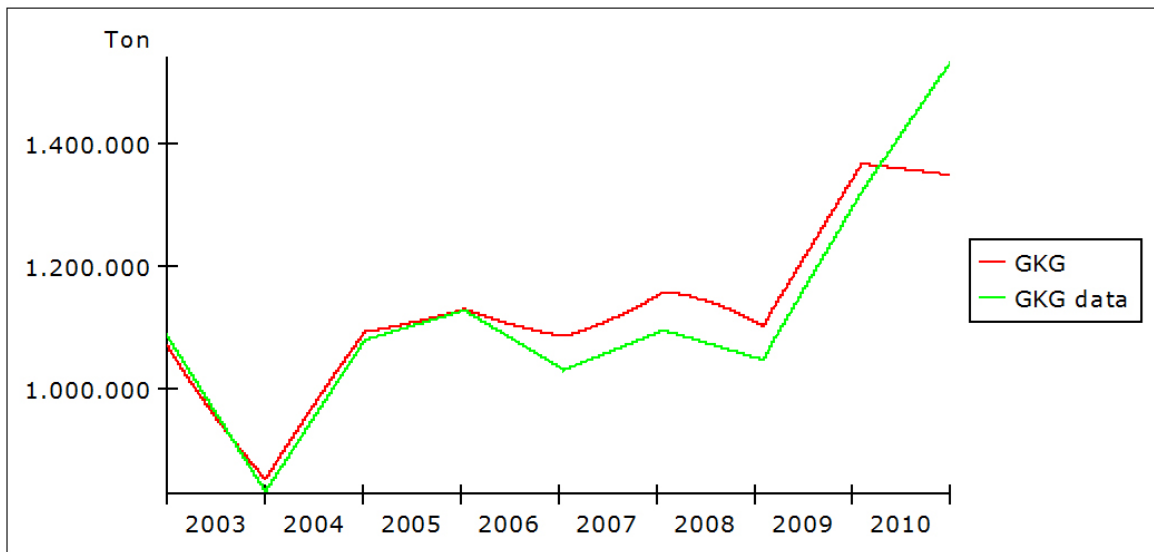
Gambar 7. Validasi model produksi GKG
