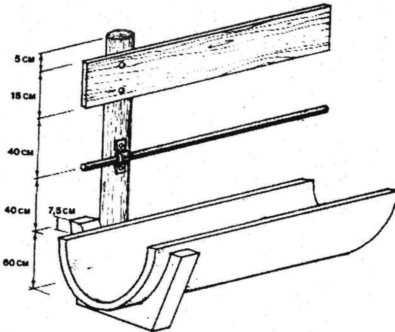
Gambar 19 Ukuran depan kandang pembesaran
