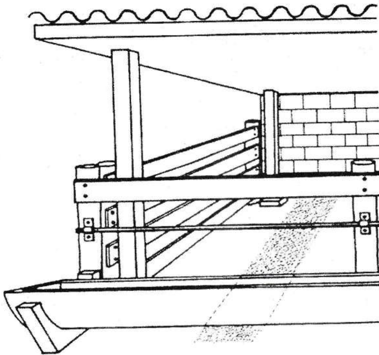
Gambar 18. Kandang pembesaran tampak dari depan
