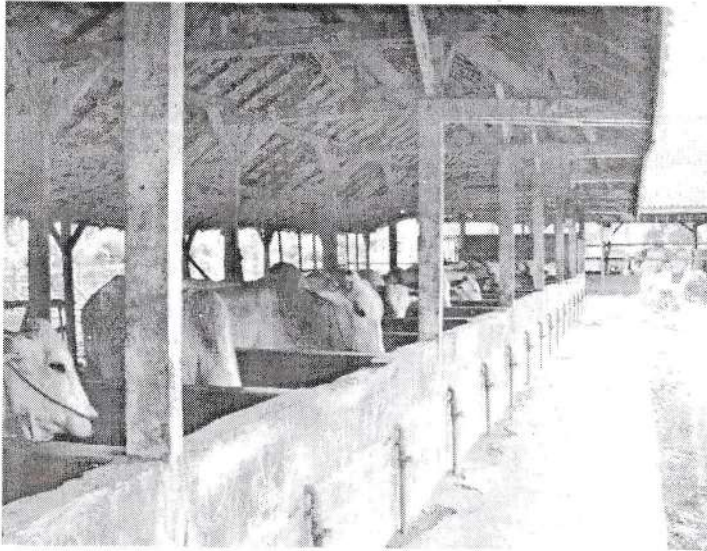
Gambar 8. Kandang individu satu baris searah tampak dari samping depan
