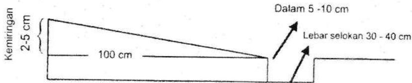
Gambar 1. Kemiringan lantai kandang dan ukuran selokan.
