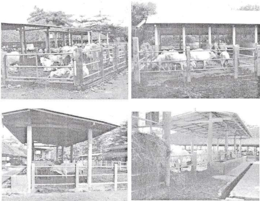
Gambar 13. Kandang kelompok beratap sebagian beserta rak penyimpanan pakan
