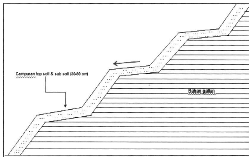
Gambar 3a. Sketsa cara penimbunan dengan bidang olah yang miring ke luar (ke arah lereng makro) menyebabkan erosi cukup besar di bidang olah dan tampungan teras (Sumber: modifikasi dari Umar 1986 dalam Puslittanak 1995)
