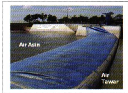
Gambar 6. Bendungan karet sebagai penghambat intrusi air laut. (Foto: Deddy Erfandi).
