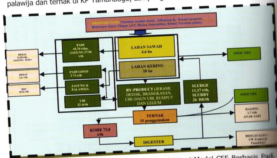
Gambar 3. Diagram Alir Pilot Plan Sistem Usaha tani Model CEF Berbasis Padi, Palawija dan Ternak di Kebun Percobaan Tamanbogo, Lampung Timur (BBSLDP 2011)
