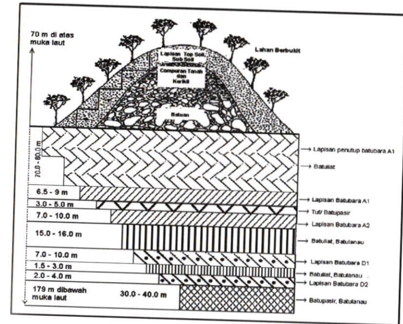
Gambar 2. Penampang galian dari puncak bukit sampai lapisan di bawah deposit batubara (Sumber: modifikasi dari Umar 1986 dalam Puslittanak 1995)
