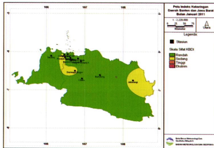
Gambar 1. Peta Indeks Kekeringan Daerah Banten dan Jawa Barat Bulan Januari 2011 ( http://www.bmkg.go.id/ImagesData/ImagesDataBW2/indekskekeringan.jpg )
