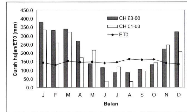
Gambar 2. Rataan curah hujan (CH) tahun 1963 – 2000 dan 2001 – 2003 serta evaporasi tahun 2001-2003 di KP Taman Bogo (Sumber: Baliittanah 2005)
