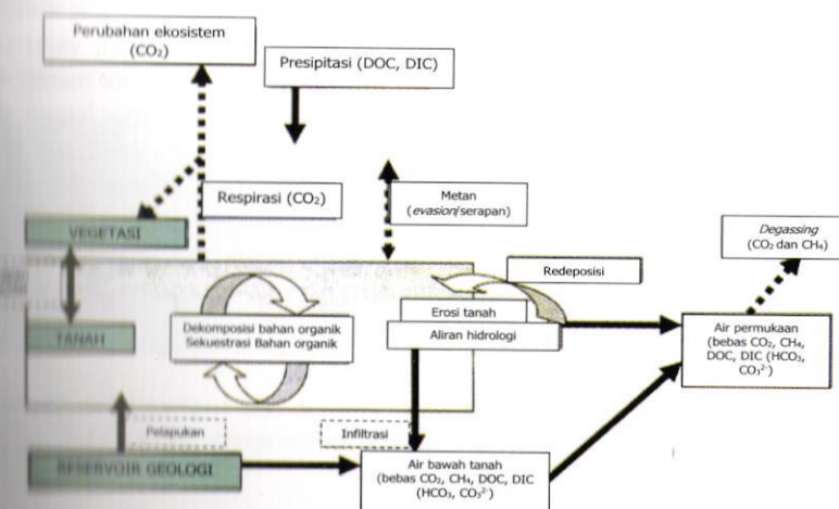
Gambar 1. Bagan alir karbon budget dalam suatu ekosistem (Billett et al. 1994 dalam Dawson dan Smitt 2007)
