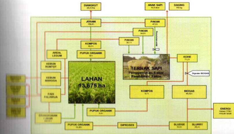
Gambar 2. Diagram alir pilot plan sistem CEF berbasis padi/palawija-ternak sapi di Kebun Percobaan (KP) Jakenan, Pati, Jawa Tengah (BBSDLP 2011)
