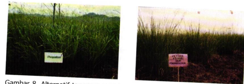
Gambar 8. Alternatif tanaman penutup tanah ( Centrosema , Calopogonium , Peuraria , Rumput Phaspalum , Rumput BD, Vetiver ) (Foto: G. Syamsidi dan S. H. Tala'ohu)
