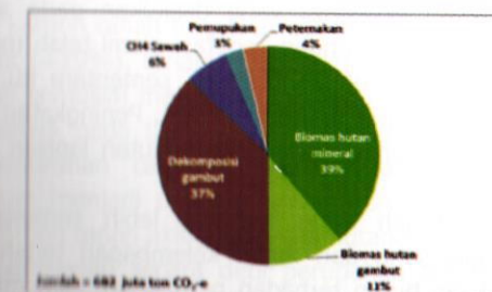
Gambar 2. Sumbangan emisi tahunan dari berbagai sub-sektor pada sektor berbasis lahan pada periode tahun dasar ( base year ) 2006-2011 (Agus et al. 2013b)
