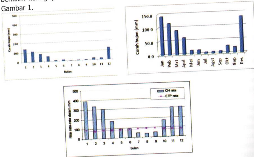
Gambar 1. Pola curah hujan di Suela, Kab. Lombok Timur, Nusa Tenggara Barat (kiri, Sudarman et al. 2010) dan Kab. Pacitan (kanan, Pujilestari et al. 2010)
