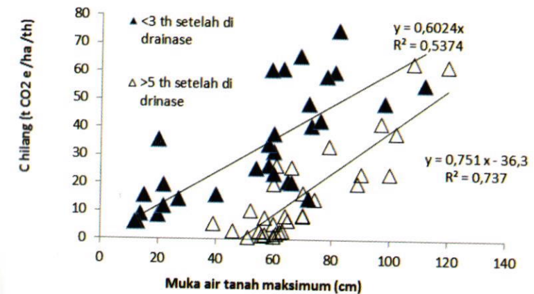
Gambar 3. Hubungan antara kondisi muka air tanah maksimum (dalam periode waktu satu tahun) dengan kehilangan/emisi karbon (Sumber data: diolah dari Maswar 2011)
