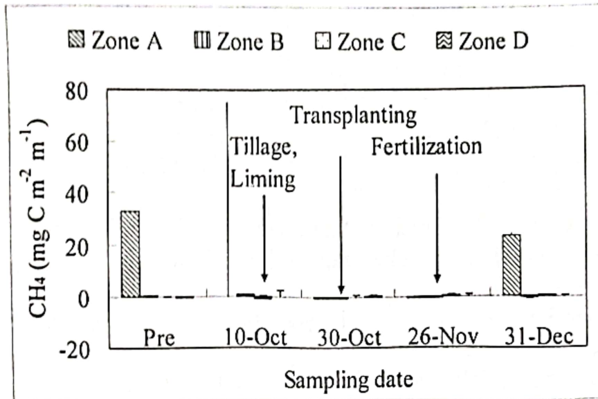
Gambar 2. Emisi CH 4 dari zone pasang surut yang berbeda pada beberapa waktu pengambilan
