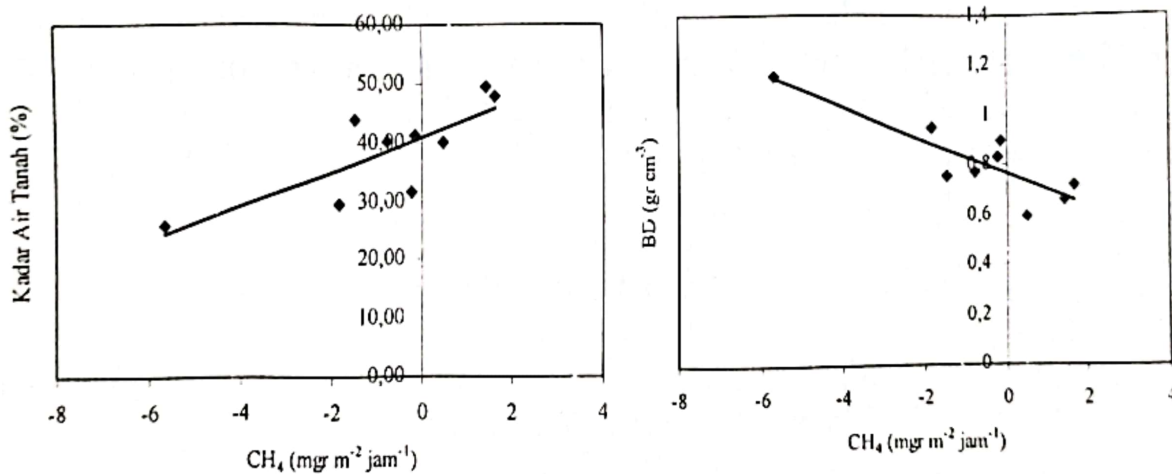
Gambar 4. Hubungan antara kadar air tanah (kiri) dan bulk density (kanan) dengan emisi CH 4 .
