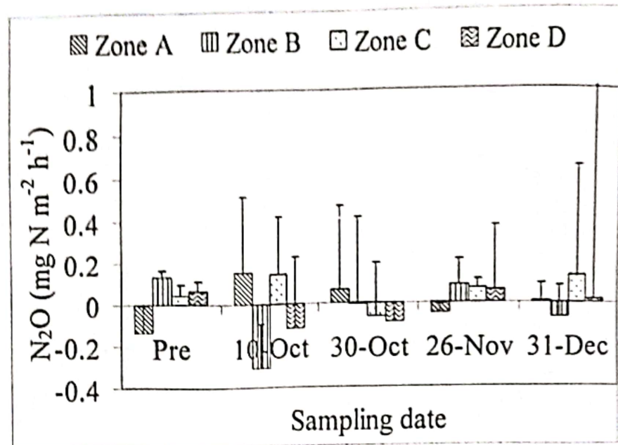
Gambar 3. Emisi N 2 O dari beberapa zone pasang surut pada beberapa waktu pengambilan
