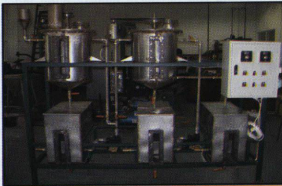
Gambar 1. Alat pengolahan Coco-Biodiesel tipe Balitka.
