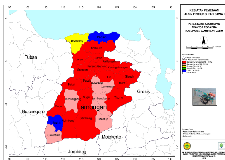
Gambar 4. Peta Status Kecukupan Traktor Roda Dua di Kabupaten Lamongan Jawa Timur (Contoh).
