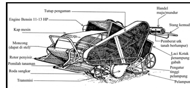
Gambar 7. Bagian-bagian mesin penyisir padi tipe SG 800
