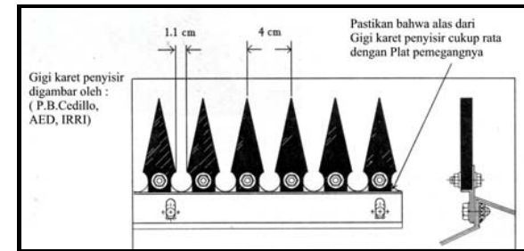
Gambar 3. Gigi penyisir menempel pada drum rotor, terbuat dari bahan ban bekas mobil
