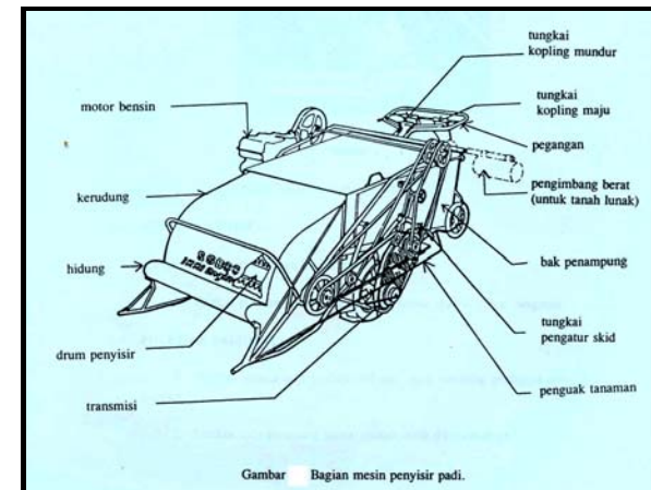
Gambar 1. Bagian mesin penyisir padi.
