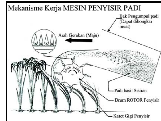
Gambar 4. Cara kerja mesin penyisir padi
