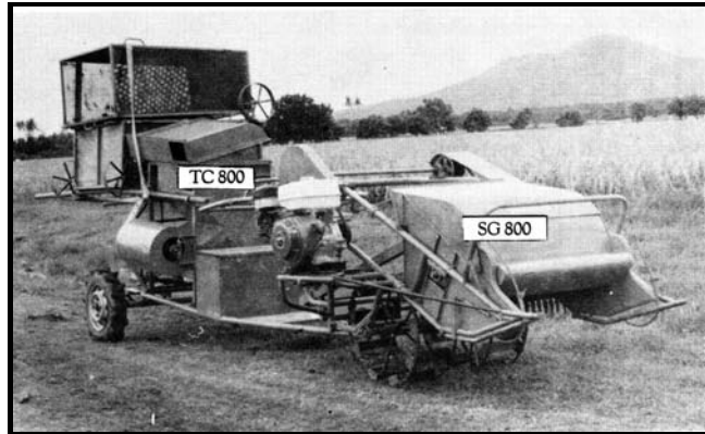
Gambar 2. Mesin penyisir padi SG 800, lengkap
