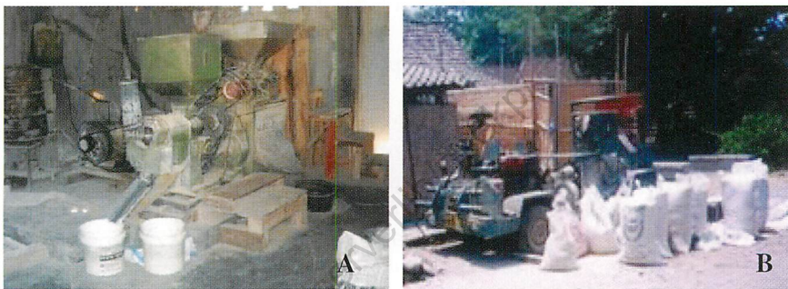
Gambar 2. Penggilingan padi skala kecil pejas giling (A) dan penggilingan padi keliling (B) (Setiawati 1999).
