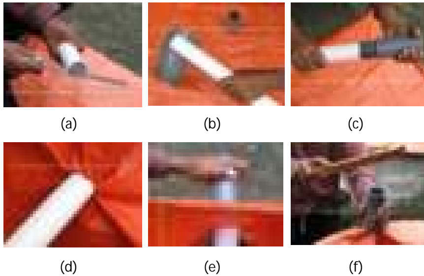
Gambar 4. Tahap Pemasangan Pralon Pembuangan Air pada Kolam Terpal
