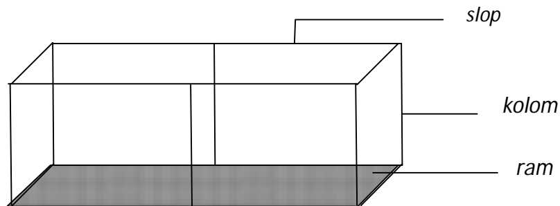
Gambar 2. Pemasangan Slop, Kolom dan Ram Sebagai Penguat Konstruksi Kolam Semen
